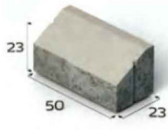
אבן שפה לאי תנועה, חצי 23\50\23
