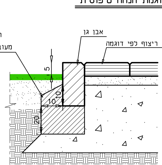
חתך טיפוסי - במפלס הריצוף
