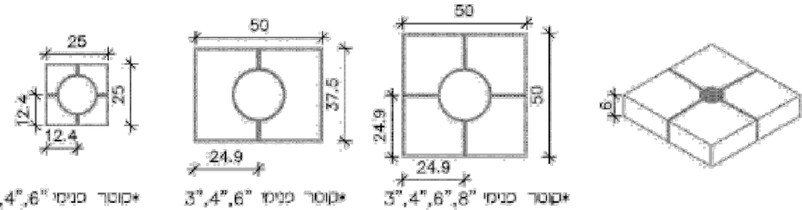
חבק סביב שני עמודים צמודים מילוי בטיט שקוע מתחת לפני הריצוף בגוון עפ"י הנחיית האדריכל
