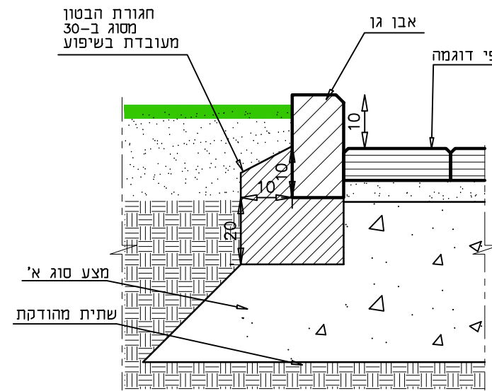
חתך טיפוסי - ערוגה מוגבהת
